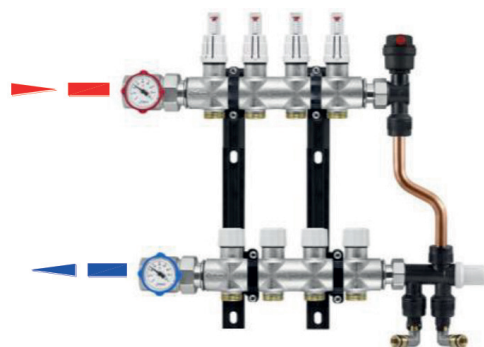
Installation correcte du collecteur avec débitmètre
